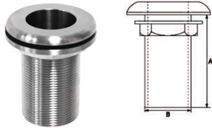
TITANIUM ALLOY THRU-HULL 钛合金全丝出水口
