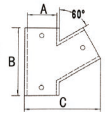
AISI316 STAINLESS STEEL 60°HANDRAIL TEE 316不锈钢 60°开口三通
