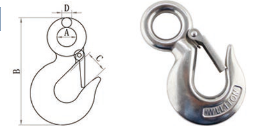
S320 CRANE HOOK S320 货钩
